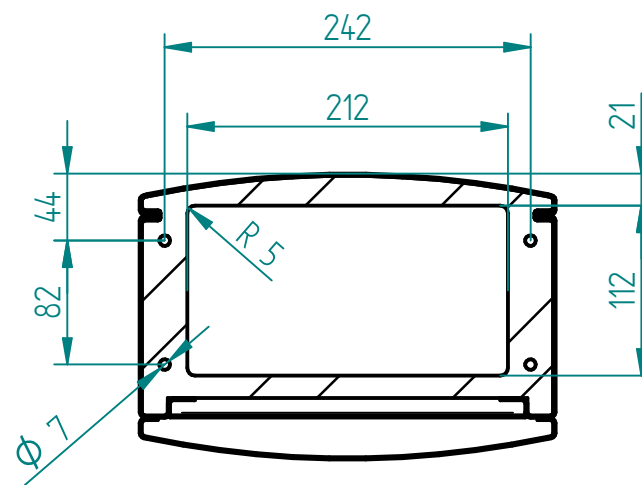
Schnitt B-B
