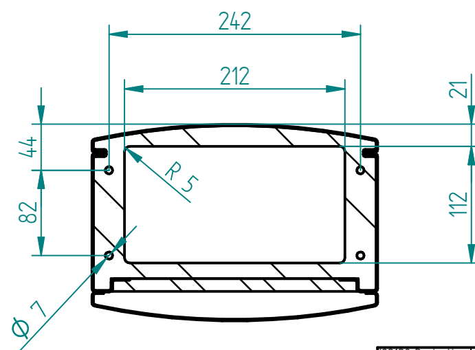
Schnitt B-B
