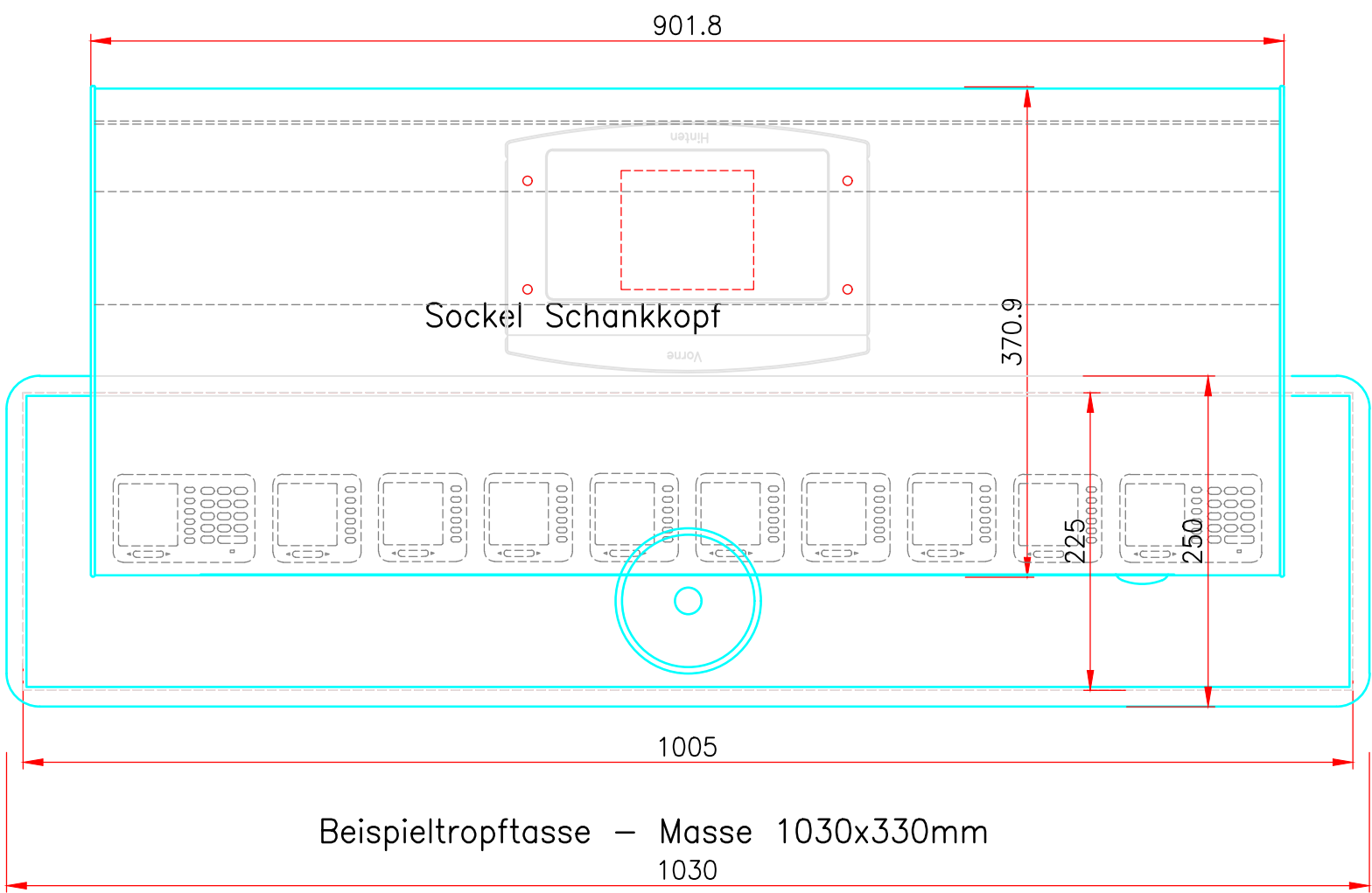
DRAUFSICHT
