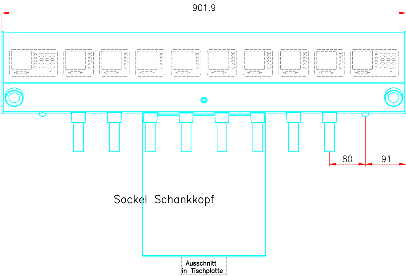
ANSICHT VORNE
