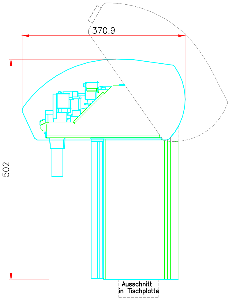
ANSICHT SEITE
